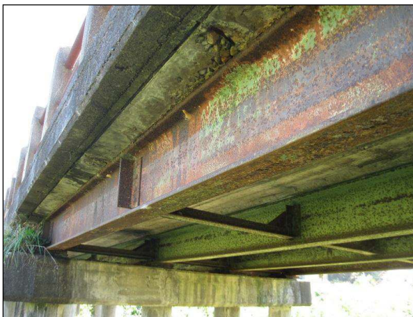
鋼桁の腐食等
